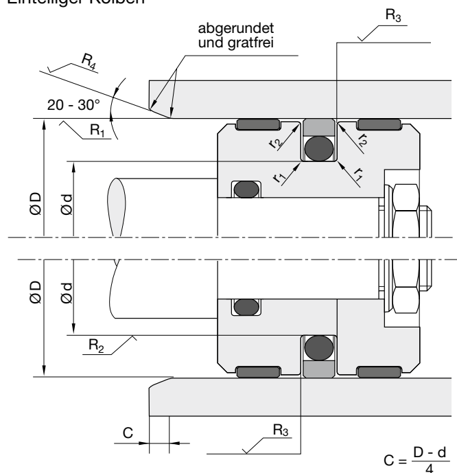
Mehrteiliger Kolben
