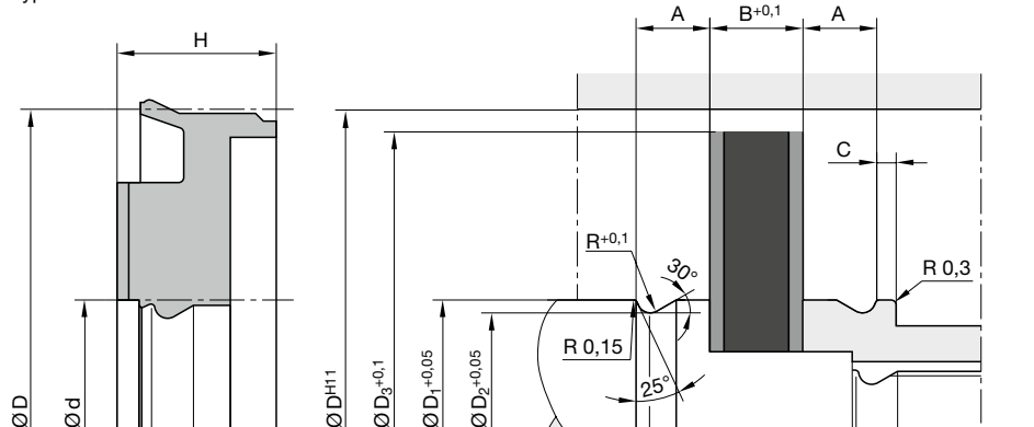
Typ 1: D < 32 \text{ mm}
