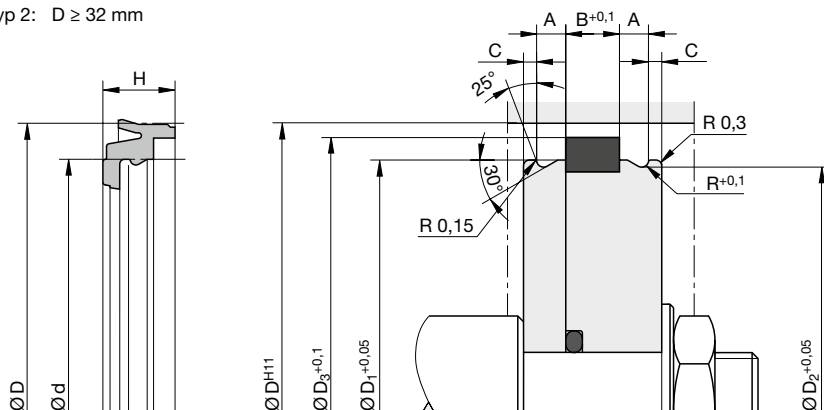
Typ 2: D \geq 32 \text{ mm}
