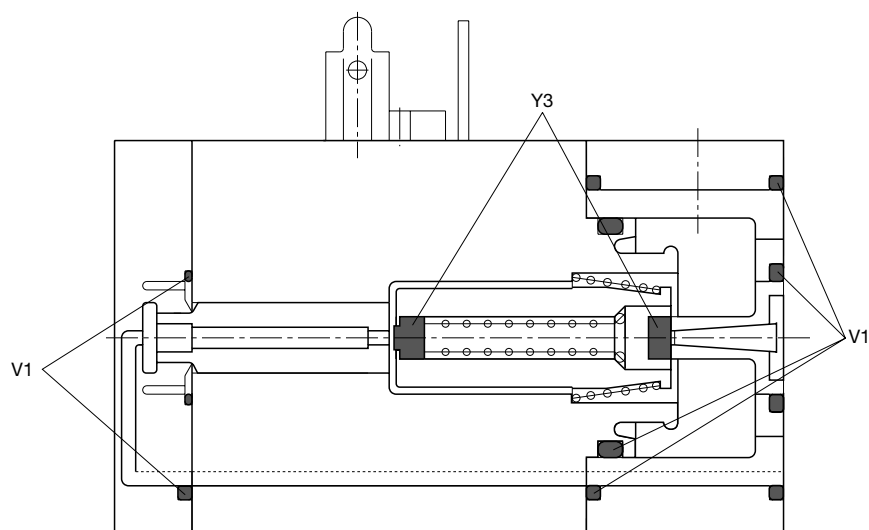
Vorsteuerventil
