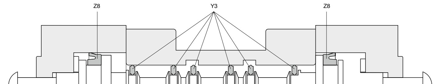
Schieberventil
