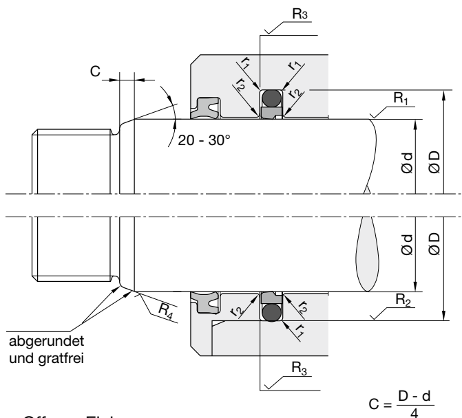
Offener Einbautraum
